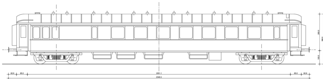
VOITURE 2976 | TAURUS
