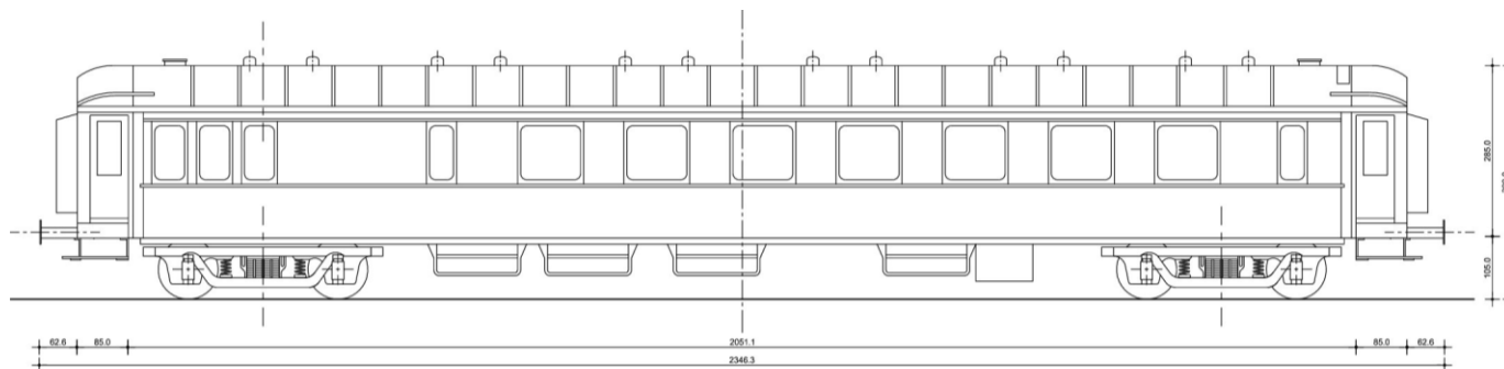
VOITURE 2976 | TAURUS
